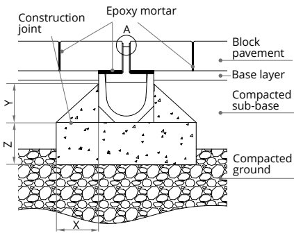
A15 - B125 - C250
