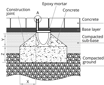
A15 - B125 - C250
